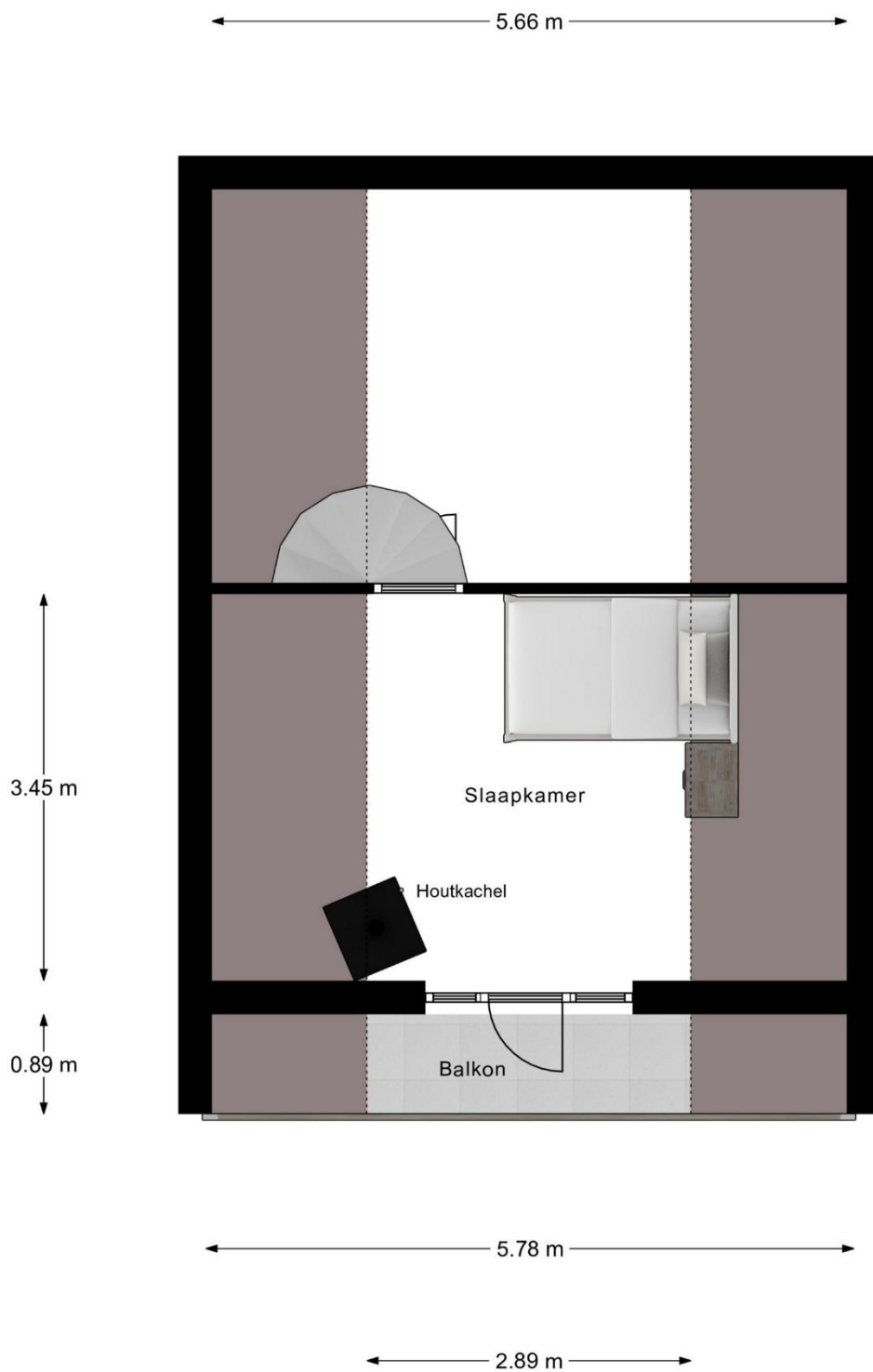
1e Verdieping
