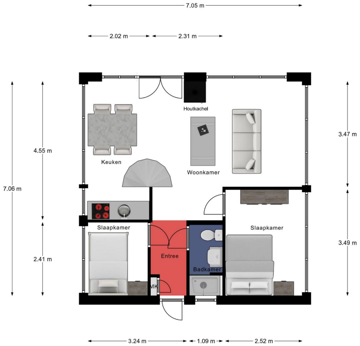
Begane Grond
